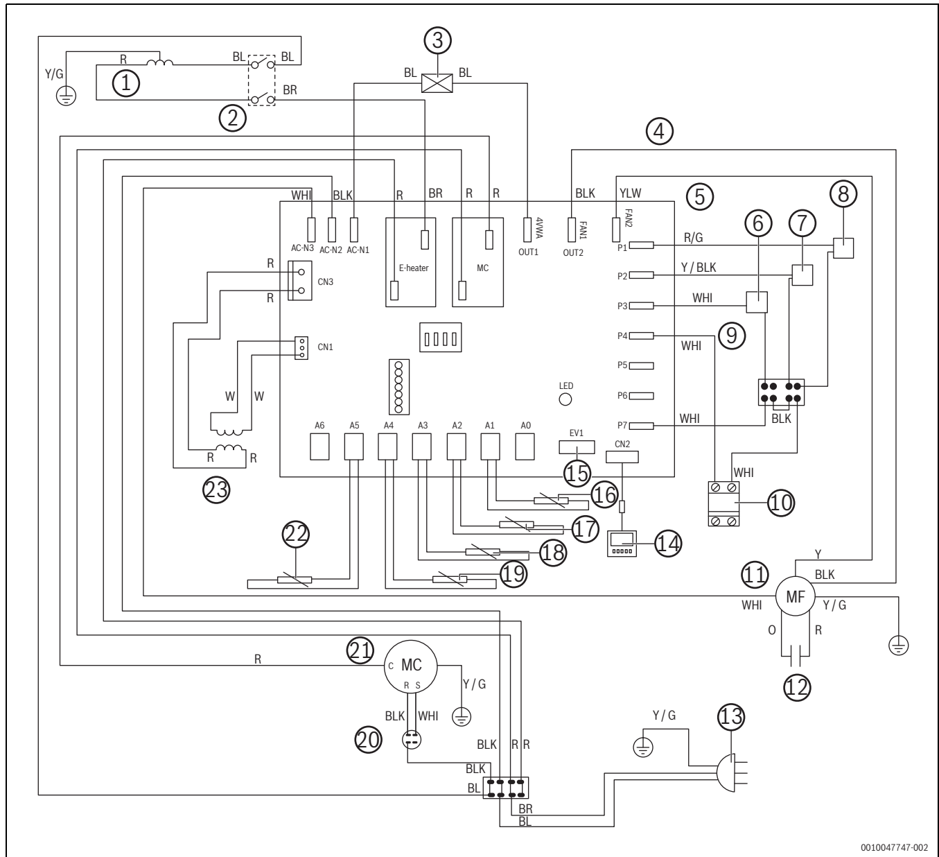
Fig. 35 Diagrama elétrico
