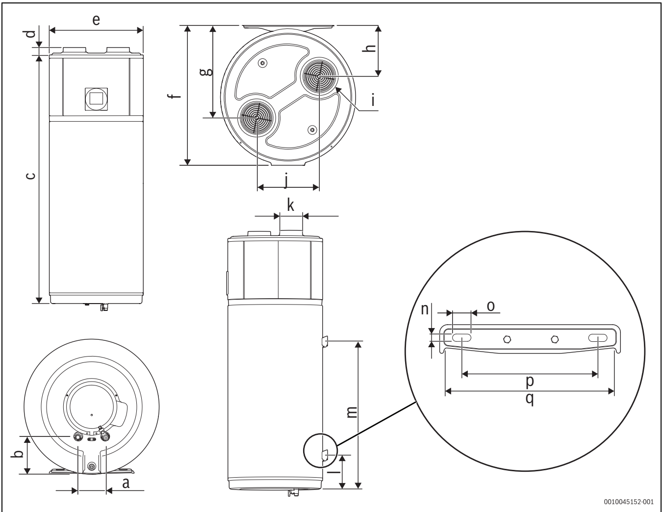
Fig. 2 Dimensões do aparelho
