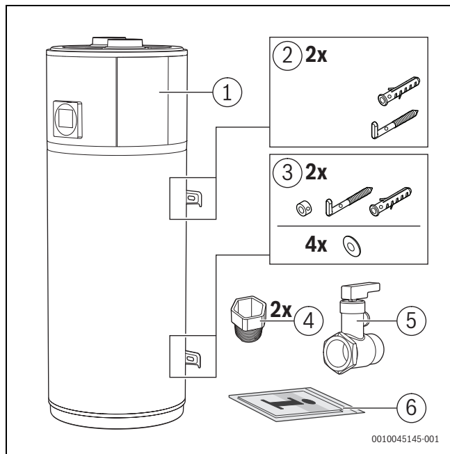
Fig. 1 Equipamento fornecido
