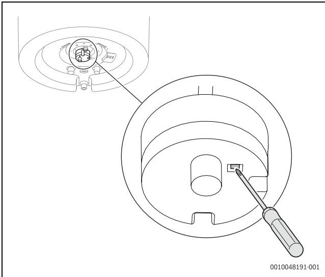
Fig. 34 Rearme do termóstato de segurança
