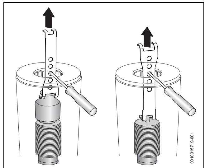
Fig. 37 Remova os defletores superior e inferior
