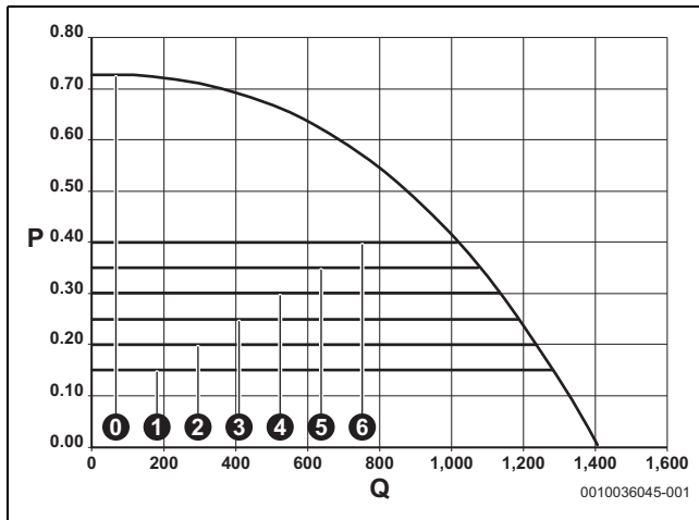
Fig. 60 Campos de funcionamento da bomba e curvas características da bomba
