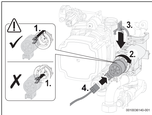
Fig. 53 Instalação do motor na válvula de 3 vias (variante sem parafusos)
