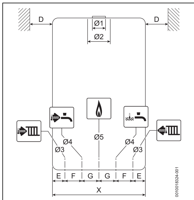
Fig. 3 Vista frontal
