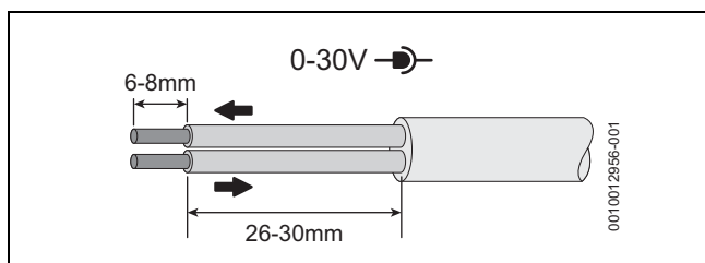
Fig. 23 Preparação para baixa tensão (cabos de sinal)
