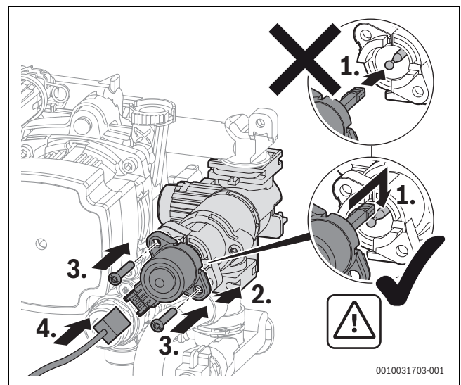
Fig. 55 Instalação do motor na válvula de 3 vias (variante com parafusos)
