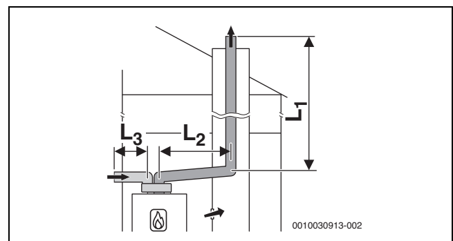
Fig. 10 Tubagem rígida de gases queimados de acordo com C 53 na condução e condução dos gases de escape para o exterior com tubos separados para ar de admissão e escoamento de gases queimados no local de instalação
