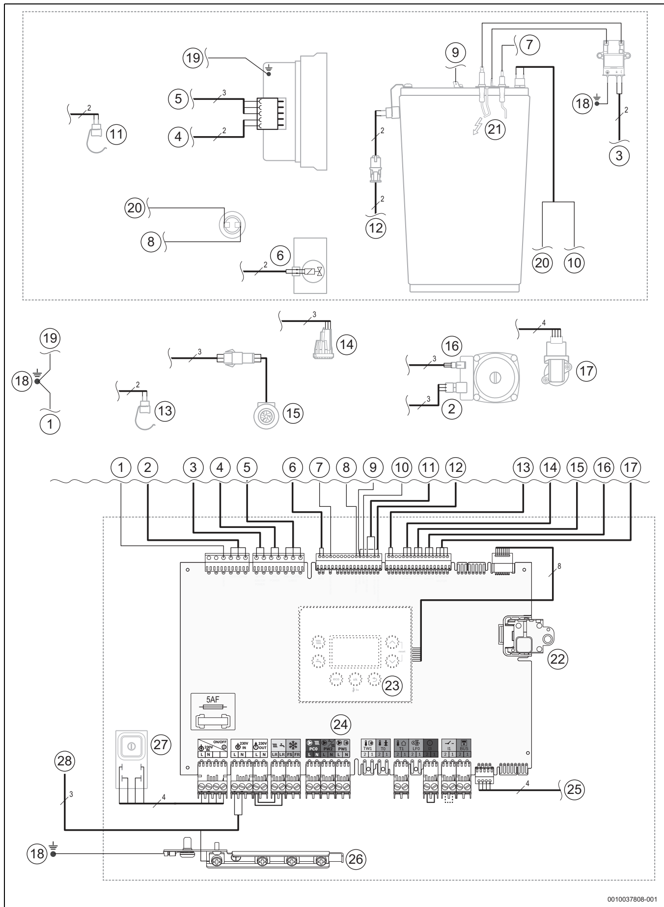
Fig. 61 Cablagem elétrica
