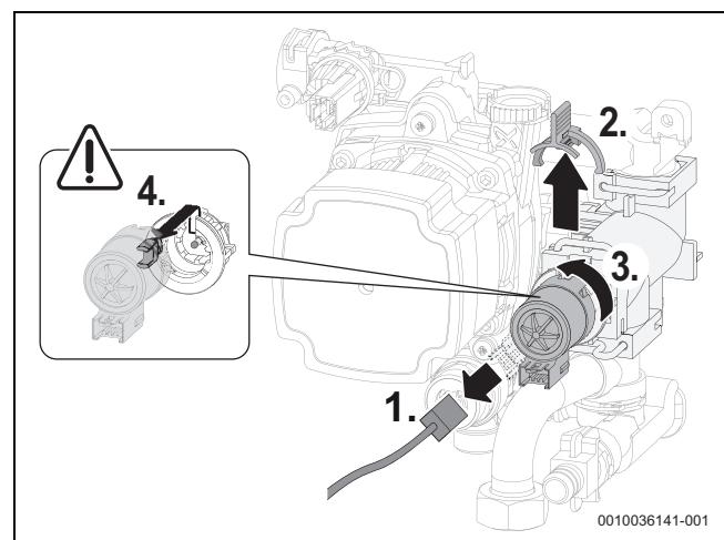
Fig. 52 Soltar o motor da válvula de 3 vias (variante sem parafusos)
