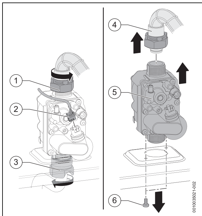
Fig. 51 Remoção da válvula de gás
