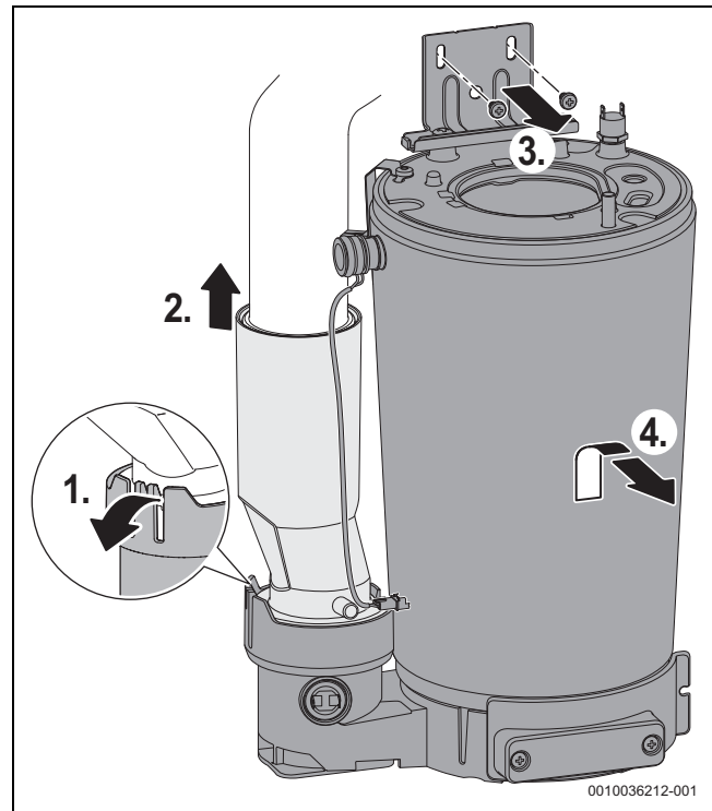
Fig. 57 Desmontar o conjunto do permutador de calor
