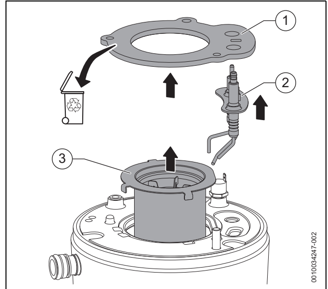
Fig. 36 Desmontar o queimador
