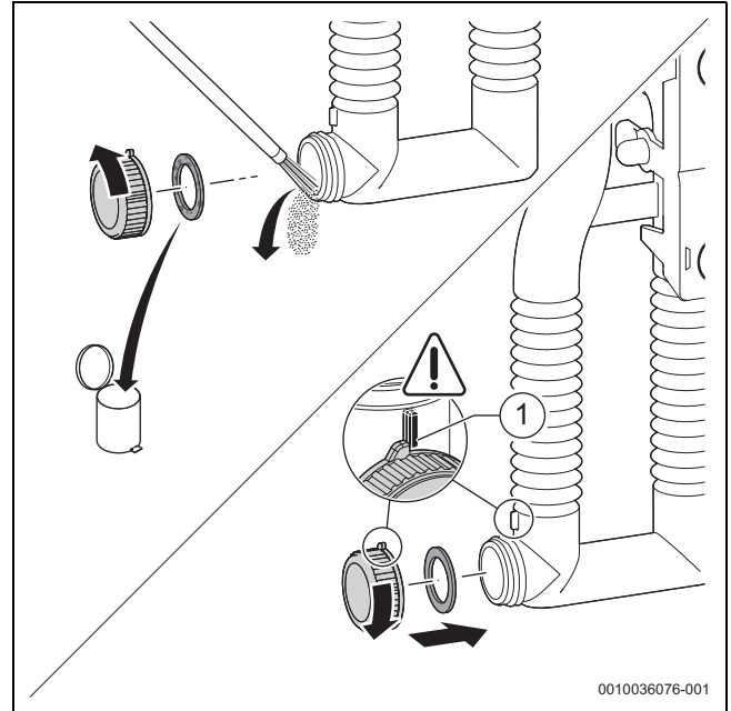
Fig. 42 Limpar a recolha de condensados
