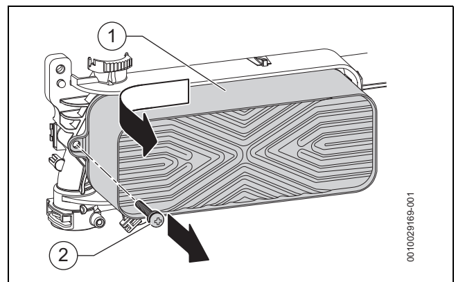
Fig. 50 Desmontar o permutador de calor de placas
