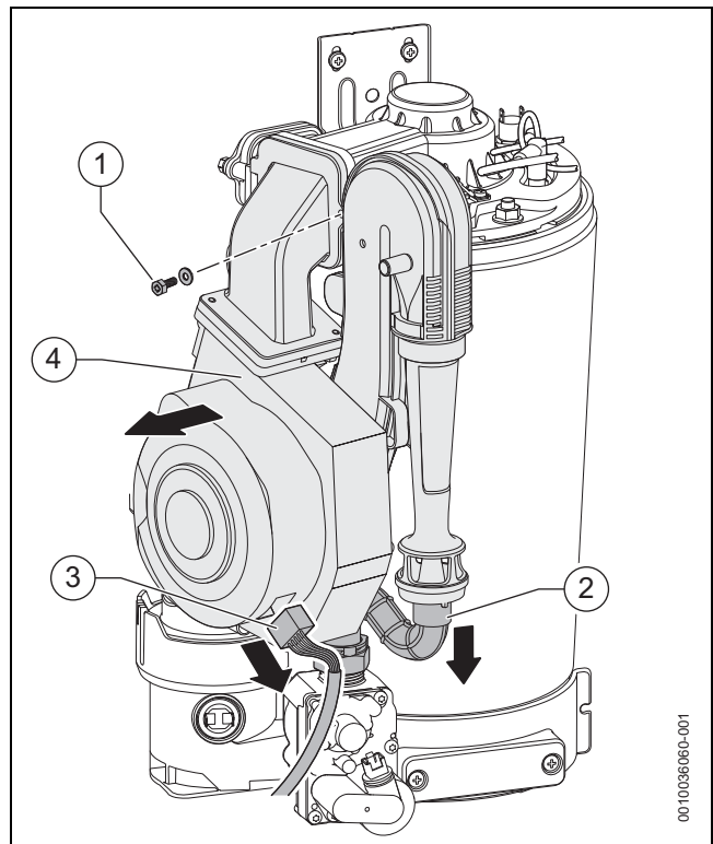
Fig. 33 Remoção do ventilador sem a unidade de mistura
