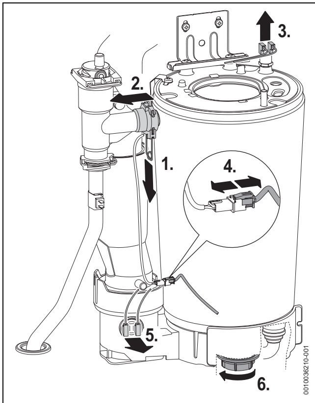
Fig. 56 Separação de componentes do conjunto do permutador de calor
