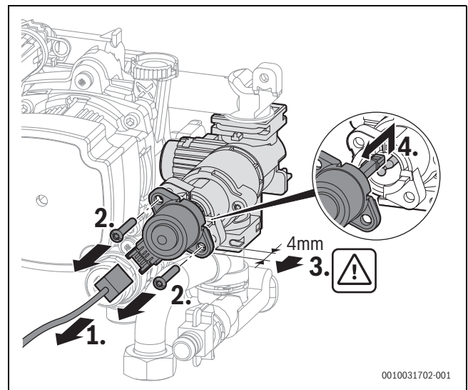
Fig. 54 Soltar o motor da válvula de 3 vias (variante com parafusos)
