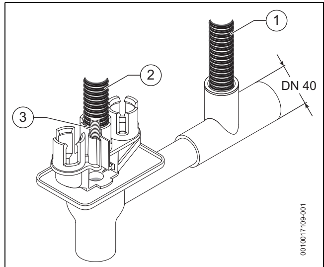
Fig. 18 Instalação das mangueiras de descarga no sifão
