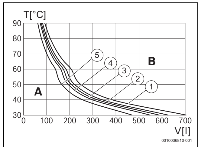
Fig. 14 Curvas características do vaso de expansão
