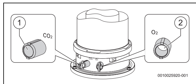
Fig. 29 Porto de medição de gases queimados e ponto de medição do ar de combustão
